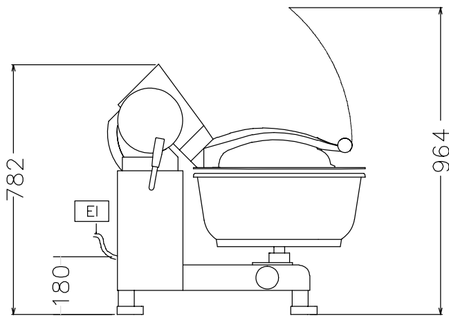
Zij aanzicht
